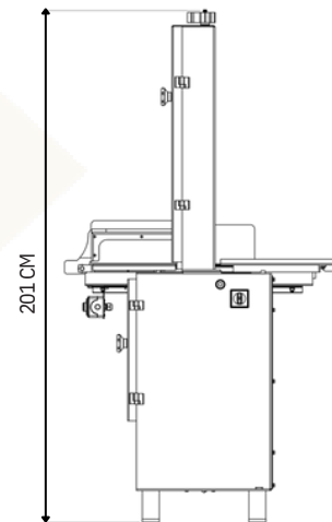
VISTA LATERAL
