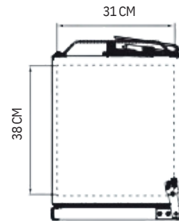
VISTA SUPERIOR
