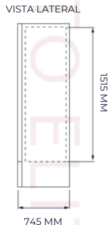
VISTA LATERAL
