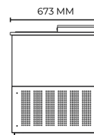
VISTA LATERAL
