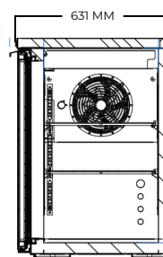
VISTA LATERAL
