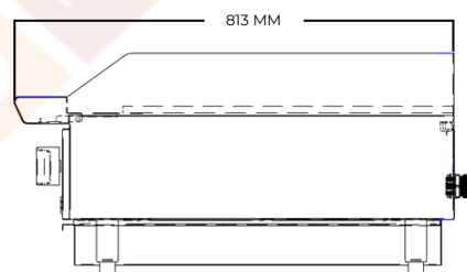
VISTA LATERAL
