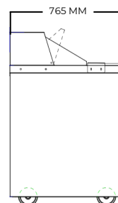
VISTA LATERAL
