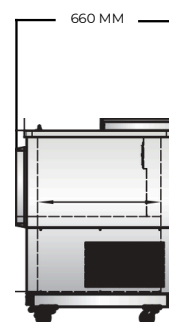
VISTA LATERAL
