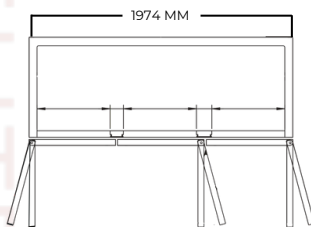
VISTA SUPERIOR
