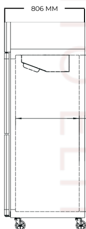
VISTA LATERAL
