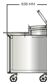
VISTA LATERAL
